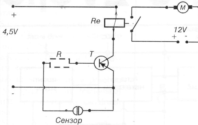
ЕЛЕКТРИЧНА ШЕМА
