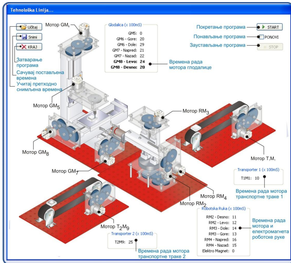
Slika 5. Izgled programa Tehnološke linije
