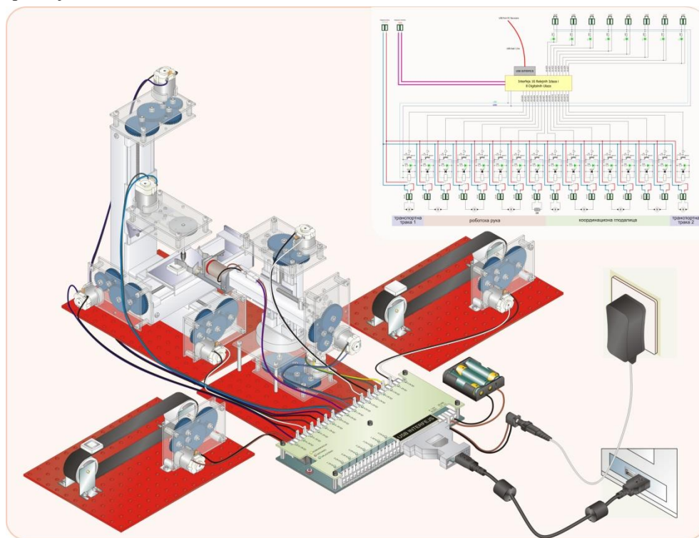
Slika 3. Model segmenta tehnološke linije sa šemom izvršnih organa
