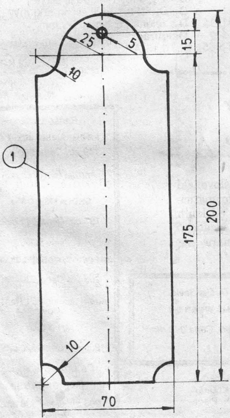
šper ploča 4x(70x200)
